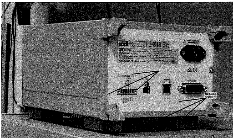
Рисунок 2 - Источник напряжения и силы постоянного тока эталонный 2553А, вид сзади
